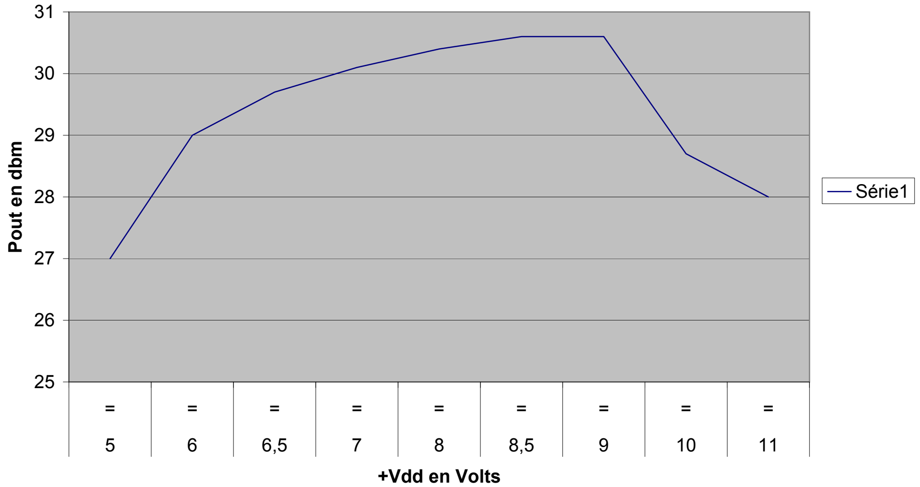
Puissance out/+Vdd, Pin=8dbm, F=10.4Ghz
